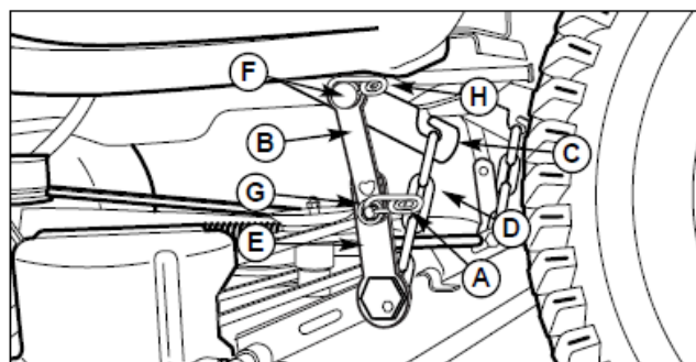
図 13 リフトアーム (トラクタの左側からの図)
