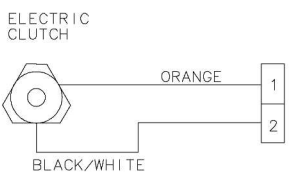
WIRING HARNESS 1726667
