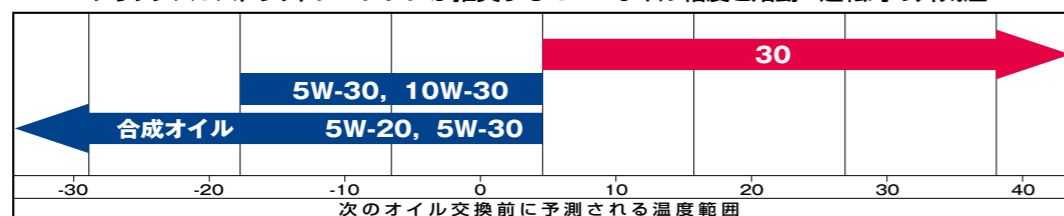
ブリッグス&ストラットンエンジンが推奨する SAE オイル粘度と始動・運転時の外気温
